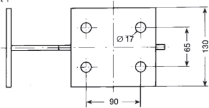
Ansicht Y
