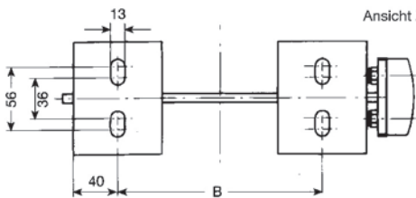
Ansicht Z
